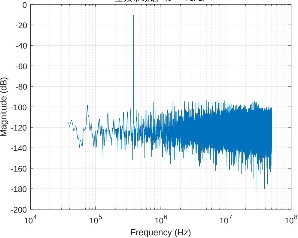
全频带频谱 (0 - f_s/2 )
